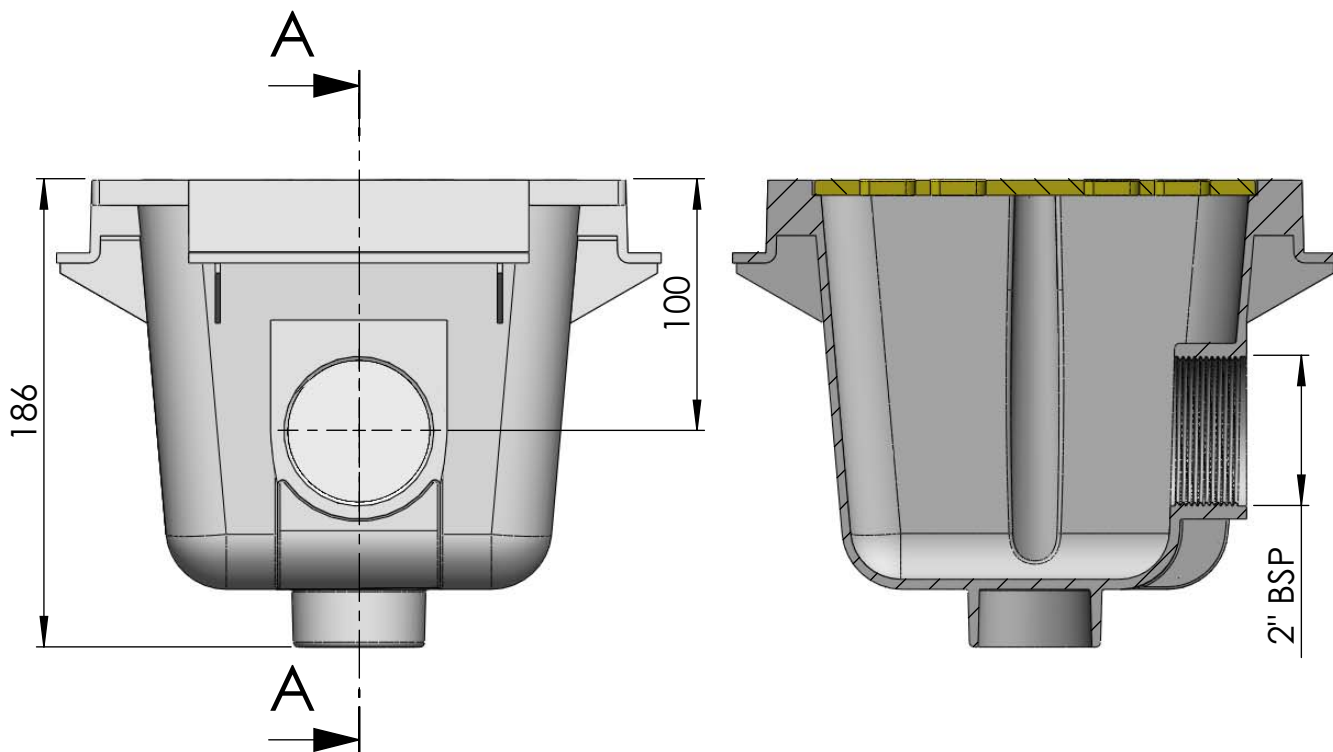
SECCIÓN A-A
