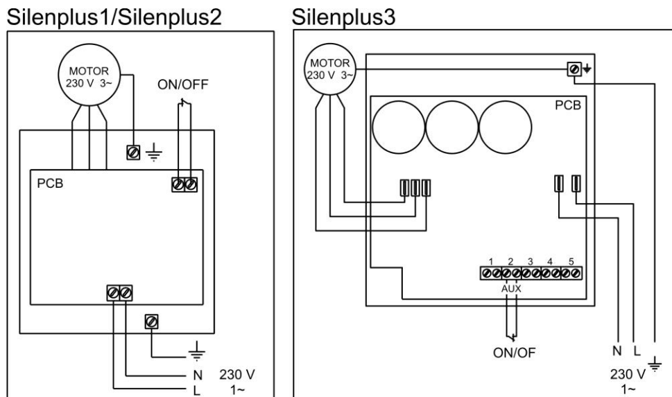
Esquema de conexiones / Connection Diagram / Schéma électrique / Schaltplan / Schema di collegamento / Aansluitschema
