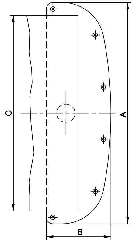
DETALLE ANCLAJE
