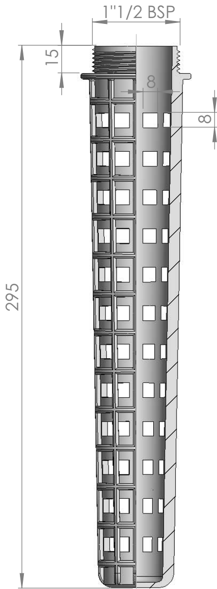
SECCIÓN A-A
