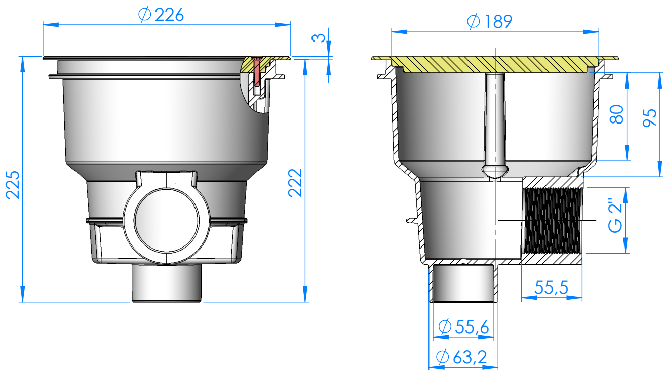
SECCIÓN A-A
